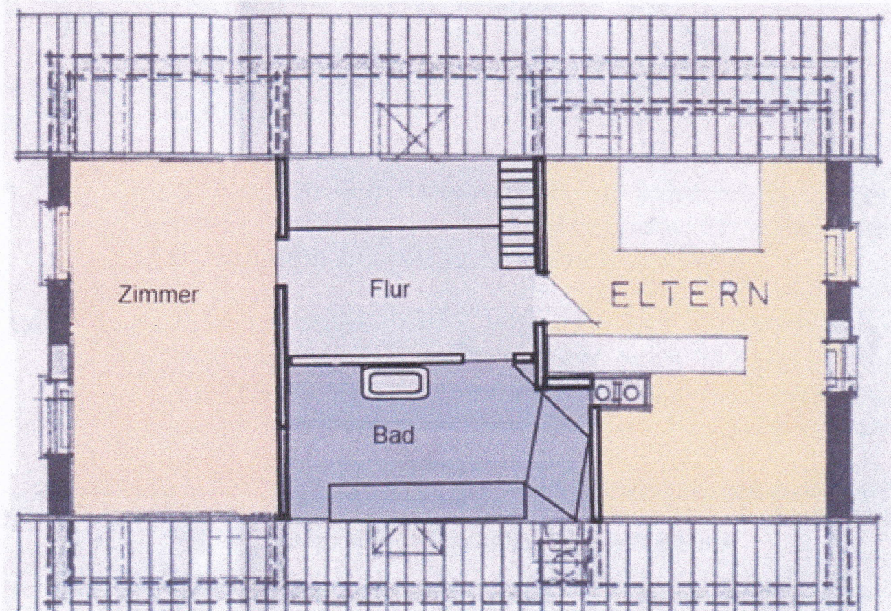
Grundriss 2.OG-Dachgeschoss
